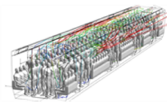
走行時の換気シミュレーション (赤、黄、緑、青の順で空気の流れが速い)
