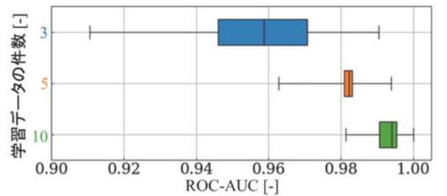
図 7 学習データの件数と提案手法の異常の判別精度
