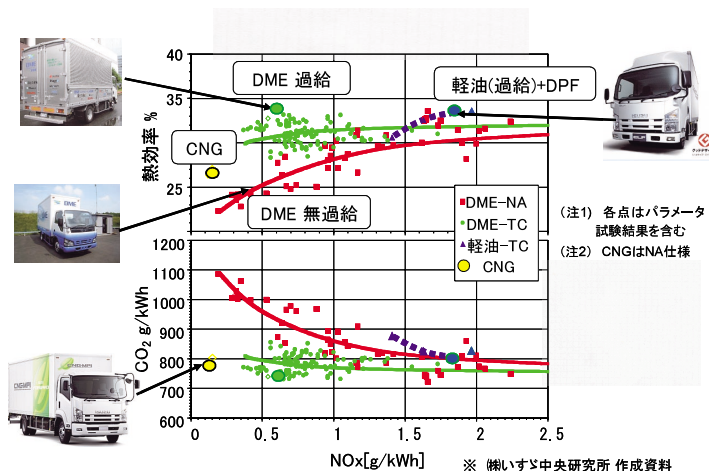
図 2 DME エンジンの CO 2 , 熱効率及び NOx（JE05 試験）
