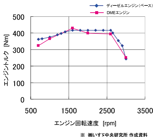
図 3 DME エンジンの出力性能
