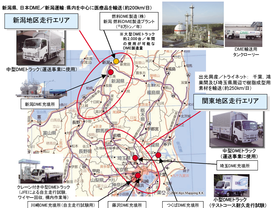
図5 実証運行モデル事業の実施地域と燃料供給・充填体制
